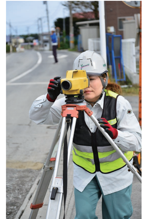
測量機器を用いて路盤の仕上げり具合を検測する笠嶋さん
